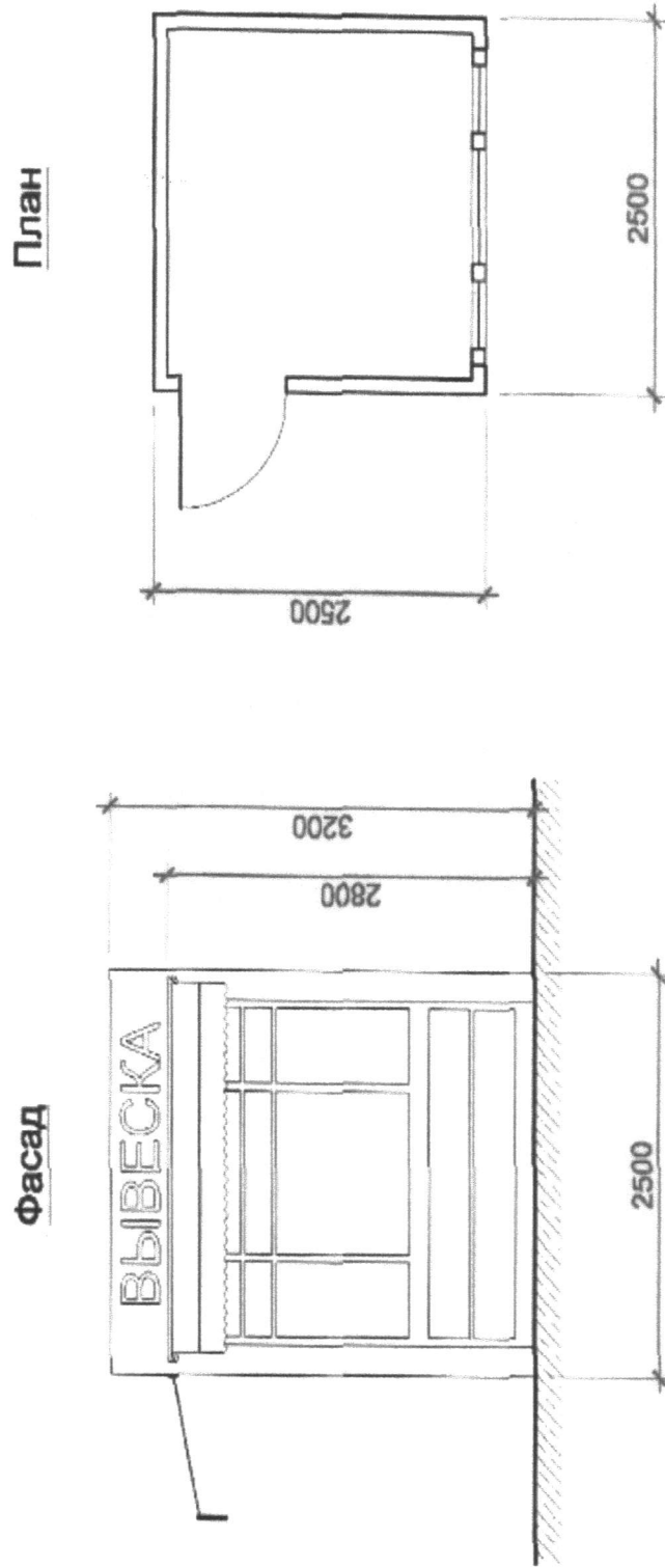
Тип 4.1. Эскиз нестационарного торгового объекта сезонного (круглогодичного) характера (прохладительные напитки, квас мороженное)
