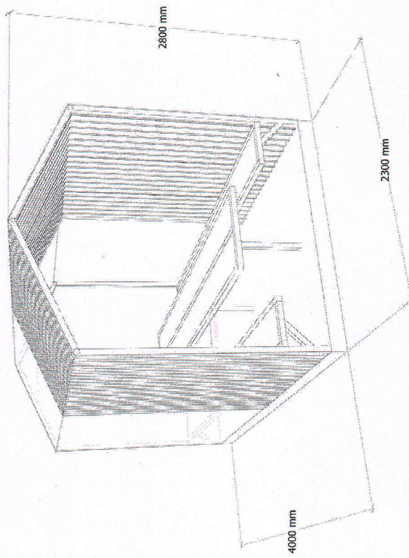
Беседка для отдыха и приема пищи
