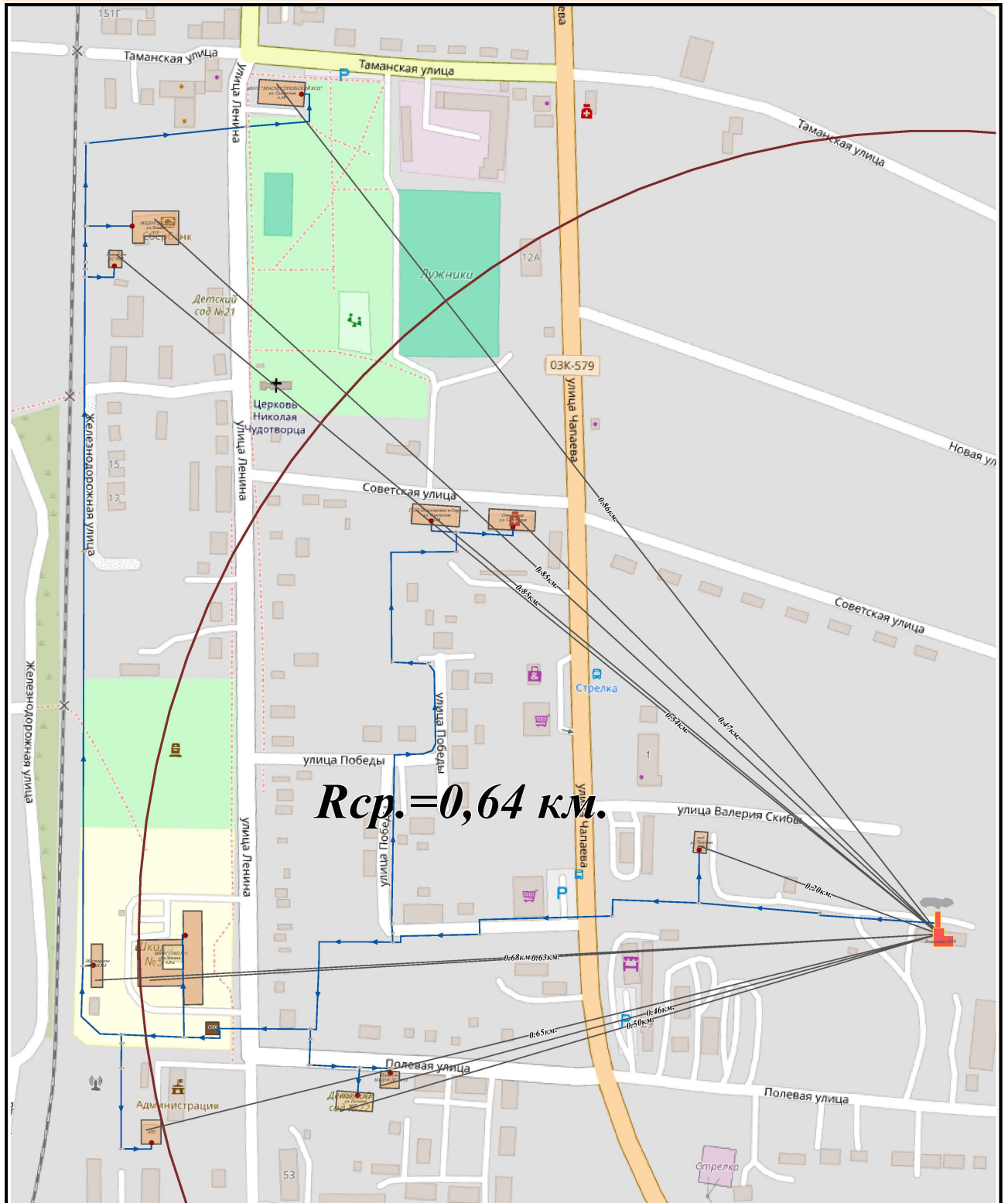
Рисунок 2.5.1 – РЭТС Котельной № 50, п. Стрелка
