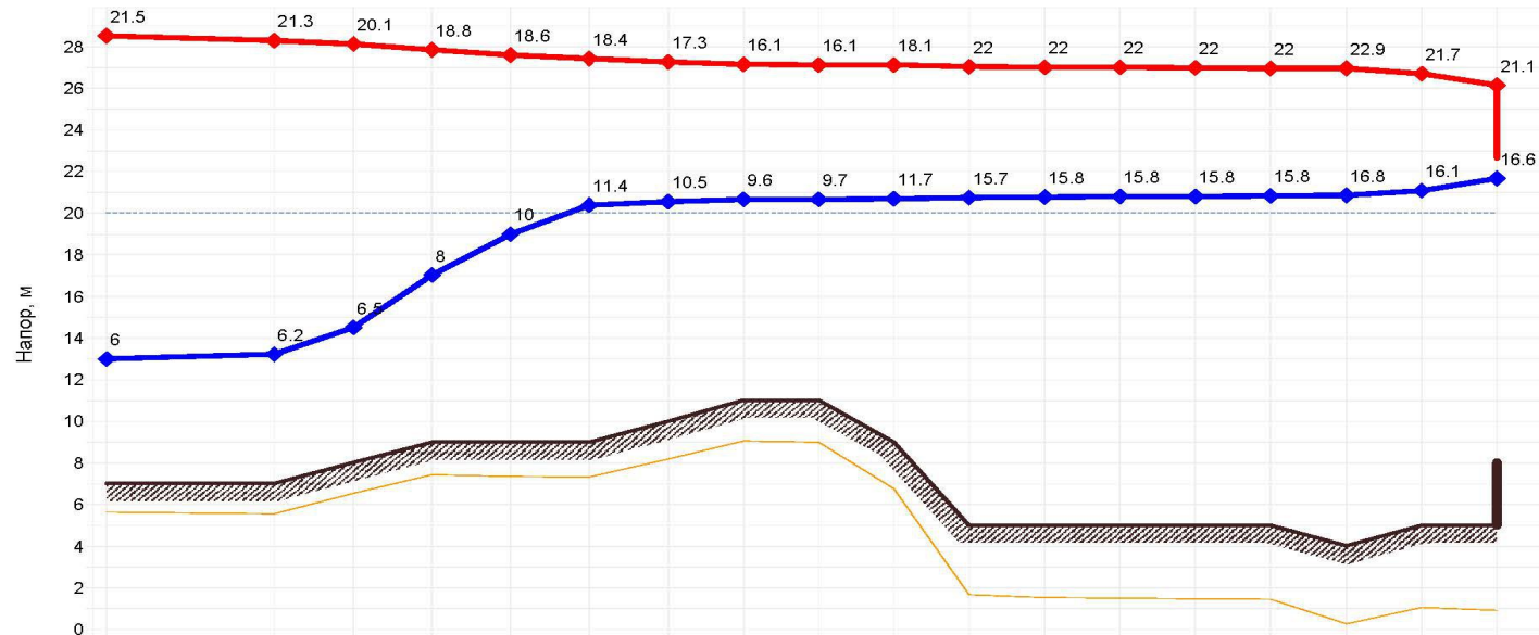
Пьезометрический график от «Котельная №50» до «МБУК "КРАСНОСТРЕЛЬСКИЙ КСЦ"»
