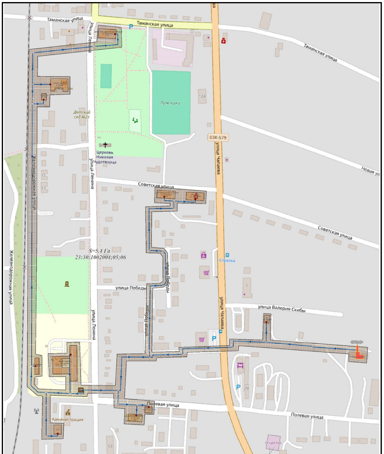
Рисунок 1.4.1 – Зона действия Котельной № 50, п. Стрелка
