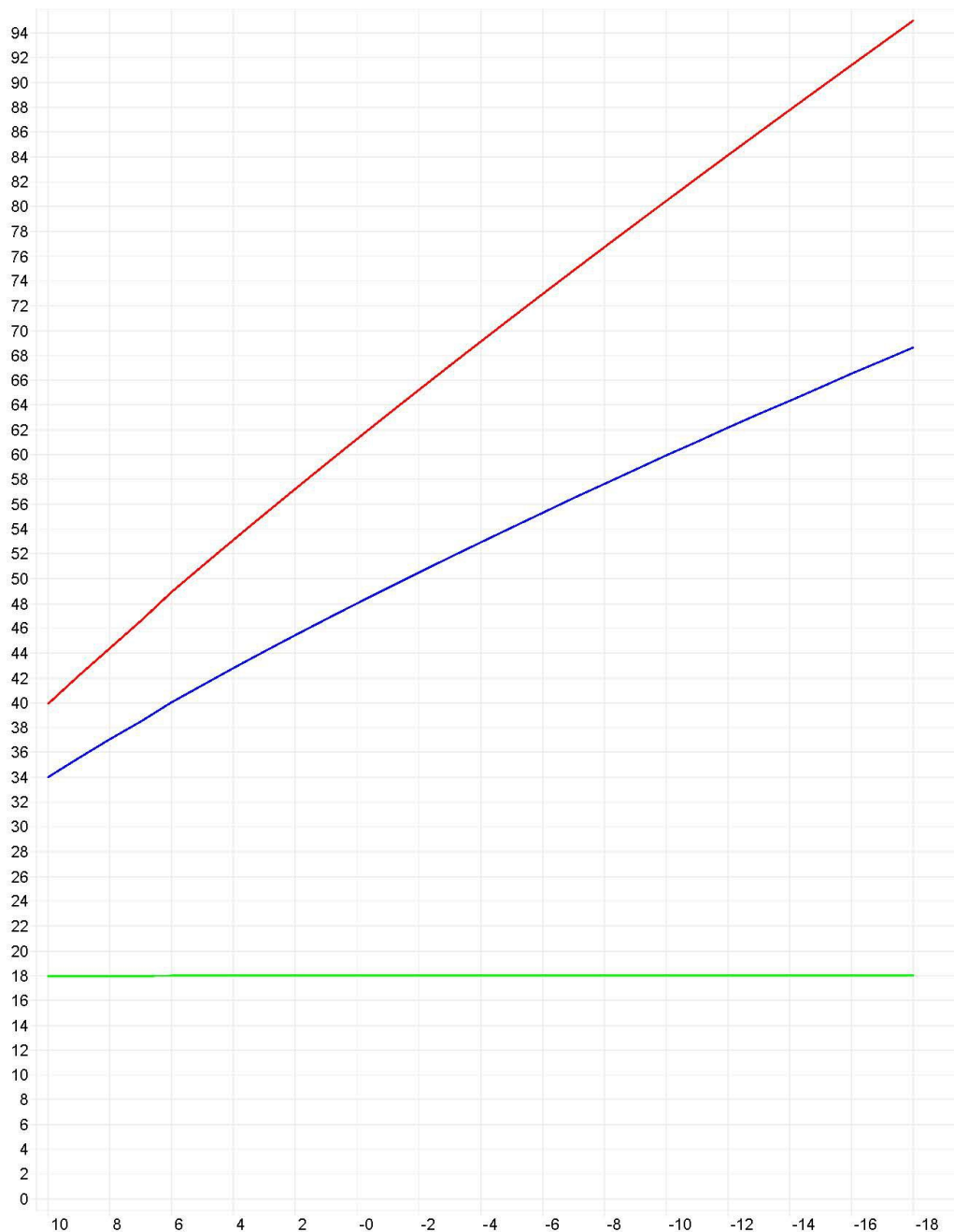
Рисунок 1.3.6.1 – Температурный график Котельных Краснострельского с. п.
