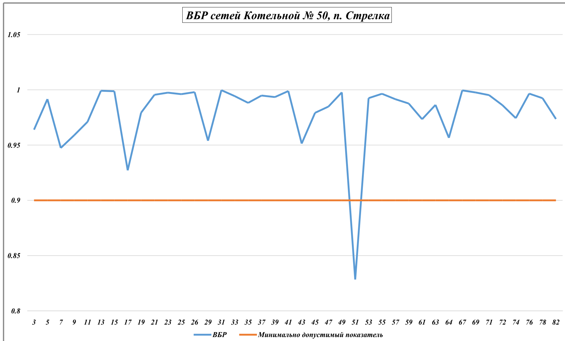
Рисунок 11.3.1 – ВБР Котельной № 50, п. Стрелка
