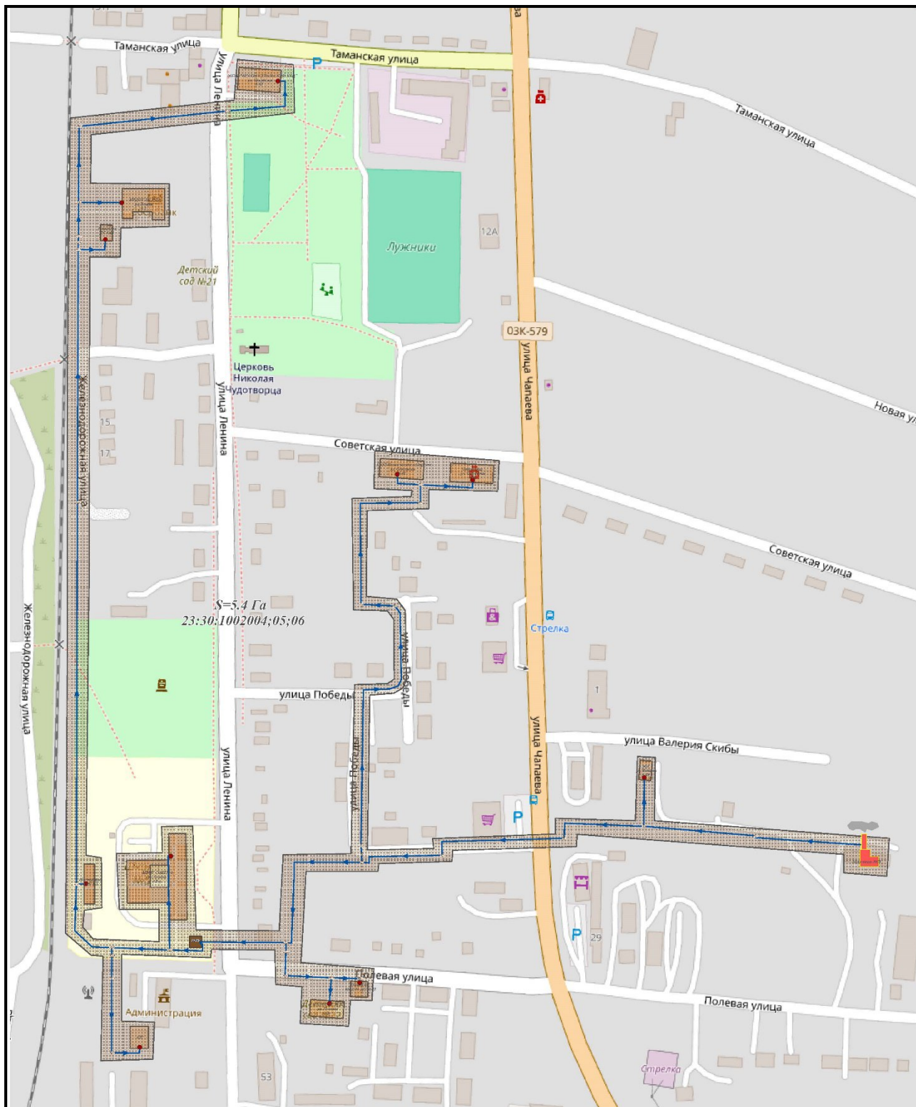
Рисунок 1.1.3.1 – Зона ТС Котельной № 50, п. Стрелка
